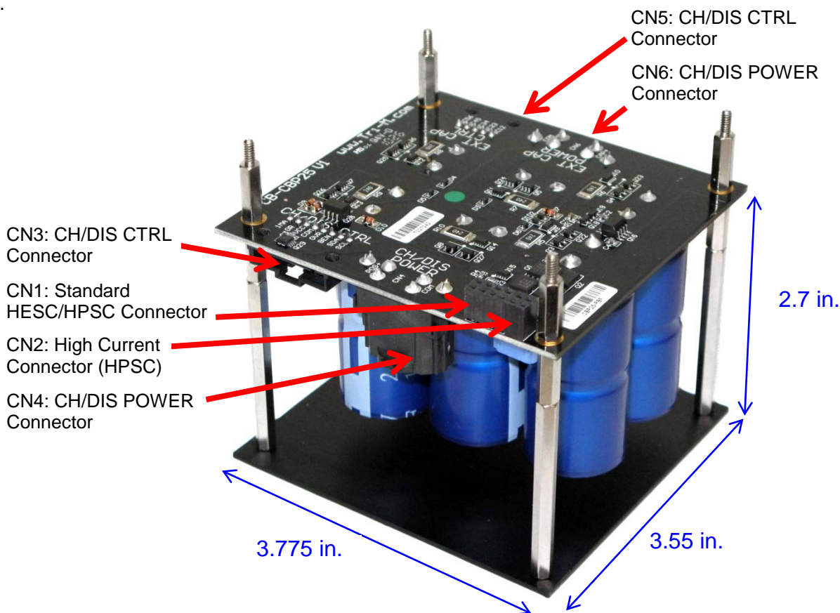
Figure 1 - CBP25-V1 Dimensions
