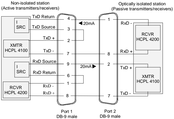
Figure 44: Current Loop wiring diagram(4 wire)
